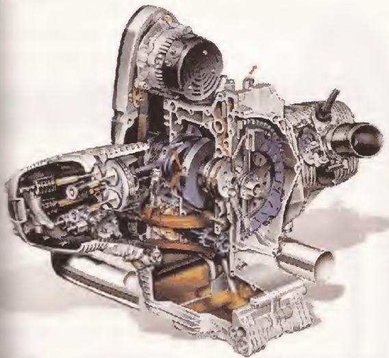
Motor en corte
